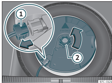
Joonis 228 Pagasiruumis: bassikõlari eemaldamine
