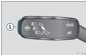
Joonis 65 Suunatulede ja kaugtulede lülituskangil: juhiabisüsteemide lüliti (sõltuvalt mudeliversioonist)
