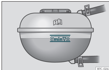
Joonis 217 Mootoriruumis: tähised jahutusvedeliku paisupaagil
