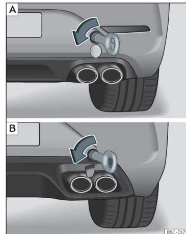
Joonis 50 Tagakaitseraua paremal poolel: sisse keeratud pukseerimisaas |A| Leon Sportstourer |B| Leon
