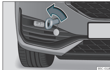
Joonis 48 Esikaitseraua paremal poolel: sisse keeratud pukseerimisaas
